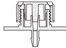
DEBİ AYARLI HAT ÜSTÜ DAMLATICI ON - LINE DRIPPERS КАПЕЛЬНИЦА С РЕГУЛИРОВКОЙ РАСХОДА قطرة
