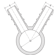
KURTAĞZI ÇOKLU DAĞITIM NİPELİ BARBED MULTICOUPLING NIPPLE РАСПРЕДЕЛИТЕЛЬНЫЙ НИППЕЛЬ РЕБРИСТЫЙ زبانه شائكة متعددة جهات
