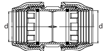
KABLİN MANŞON COUPLING МУФТА СОЕДИНИТЕЛЬНАЯ رباطة
