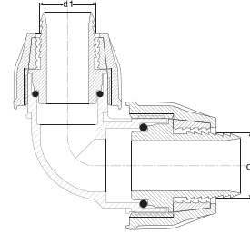
REDÜKSİYON DİRSEK REDUCING ELBOW عكس مصغرة
