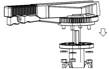
6. 180° derece döndürülmüş olan çark, kol ve kilitleme mandalı tekrar gövdeye takınız.
