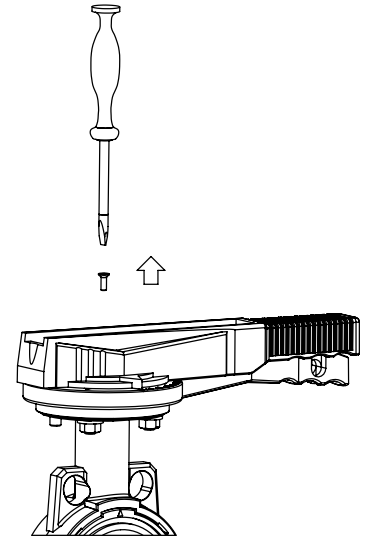
3. Tornavida yardımı ile kolu karem ile bağlayan vida sökünüz.
