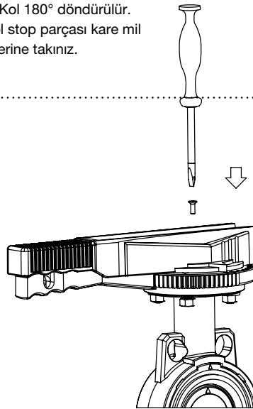
8. Kol, kare mile vida yardımı ile tutturunuz.
