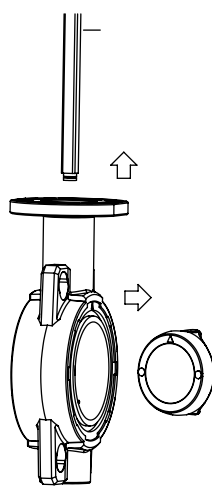
12. Kare mil dışarı çıkarıldıktan sonra klepa çıkartınız.
