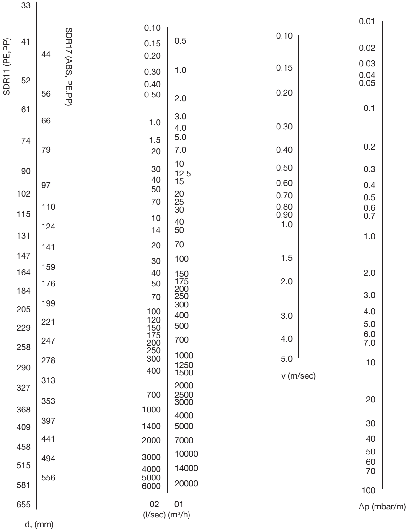
Şekil 2: Akış Nomogramı
