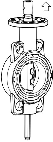
8. Kare mili 15° çevirerek vananın alt kısmından içeri sokup yukarıdaki Contalı pimi dışarı iterek çıkarınız.
