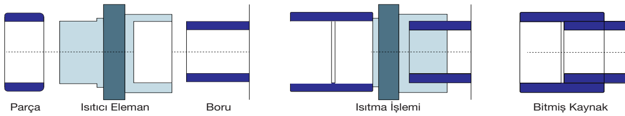
Şekil 8.2 Soket Füzyon Kaynak Tekniği
