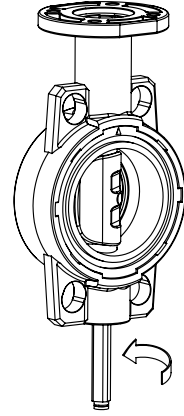
10. Aşağıdaki contalı pimi çıkarmak için kare mili 30° derece kadar döndürünüz. Kare mili ve klepayı 30° döndürünüz, kare mili tamamen vanadan çıkarınız.
