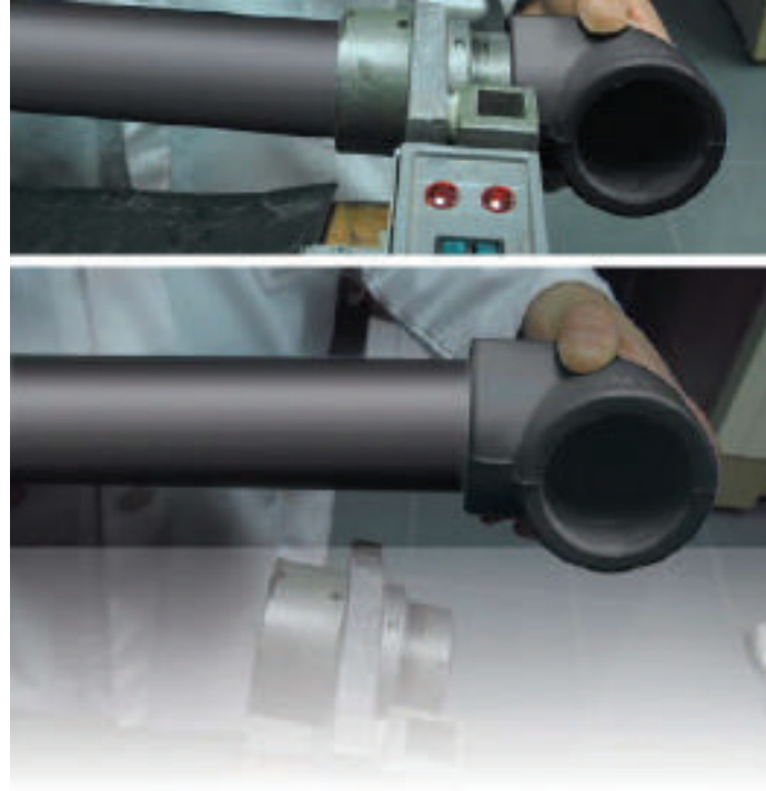
Şekil 8.2 Soket Füzyon Kaynak Tekniği
