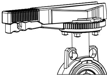
7. Klepa kapalı pozisyonda iken somunları takılarak sağlamlaştırınız.
