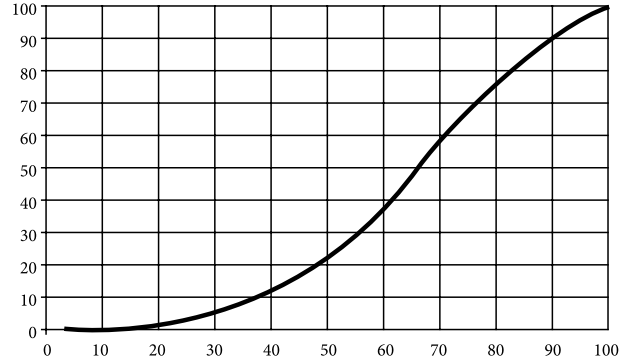
Kv % Akış Faktörü
