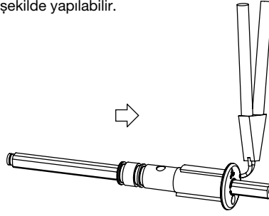
2. Stop parçası yerleştirildikten sonra segmanı takınız ve contalı pimde kare mile takınız.
