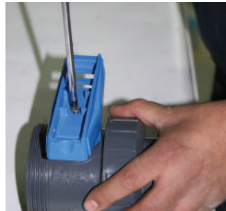
Kol üzerindeki vida yıldız uçlu bir tornavida yardımı ile sökülür.
