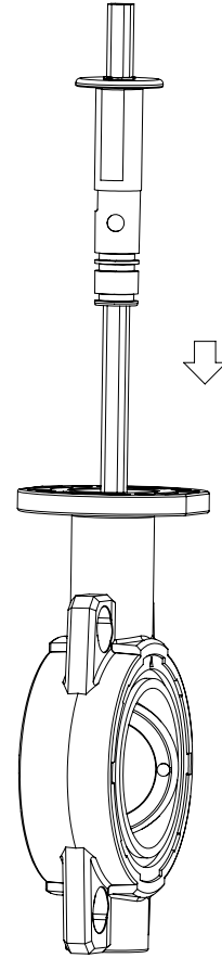
5. Kare mili yerleştiriniz ve limite kadar itiniz. Kare milin kesitine dikkat ediniz. Kare mil üzerindeki çentikleri klepa deliğindekiyle aynı pozisyonda olduğuna dikkat ediniz. Yanlış bir montajı önlemek için çentiklerden ikisi daha büyüktür.
